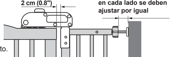
Figura 4 Aproximadamente 2 cm (0.8")
